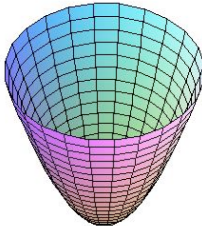
Hiperboloide x^2 + y^2 - t^2 = -1
